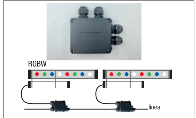
Cod. XPG9-P104 Accessorio IP67 per linee di luce continua IP67 accessory for continuous light lines.
