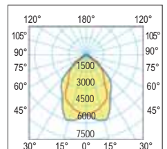
90° Diffondente - Wide
