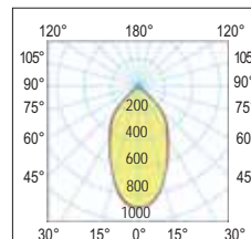
60° Semi-diffondente - Flood
