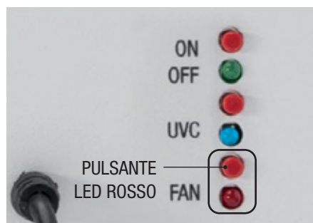
Foto 2: con il terzo tasto in basso si può modificare la velocità delle ventole, dal 100% al 50%, funzionamento al 50%, il Led rosso è acceso.
