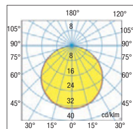
Dati fotometrici Photometric data
