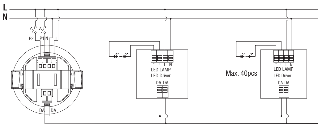
Schema di collegamento - Wiring diagram
