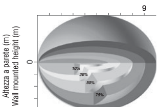
Schema di rilevamento montato a parete (m) Wall mounted detection diagram (m)
