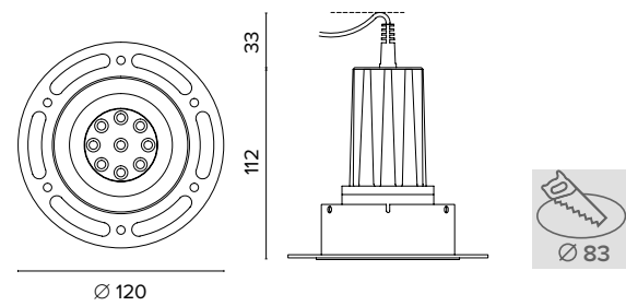
0698 SL /A tondo / round
