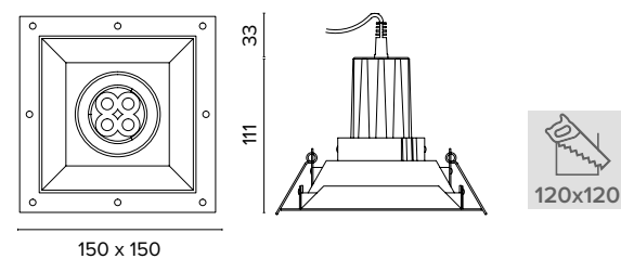
0697 SL / A quadrato / square
